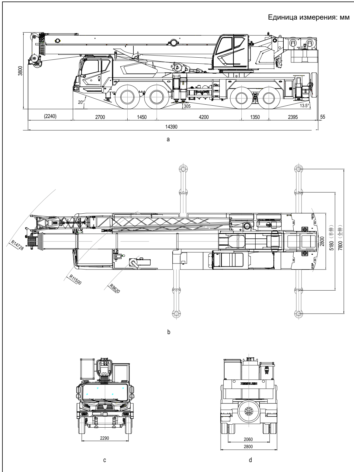
Рисунок 1-10 Габаритные размеры
