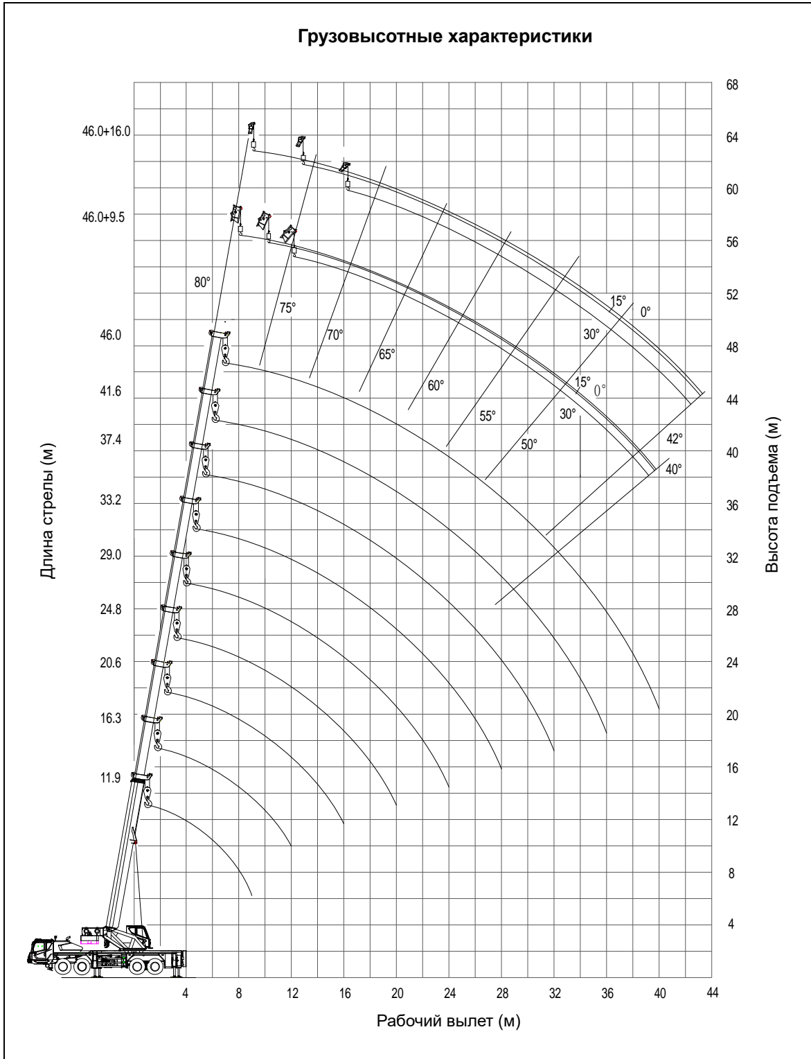
Рисунок 1-12 Диаграмма грузовысотных характеристик
